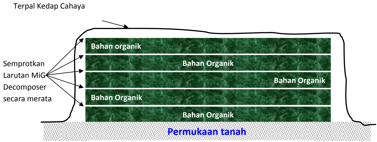
Gambar. Susunan bahan organik pada pembuatan kompos
